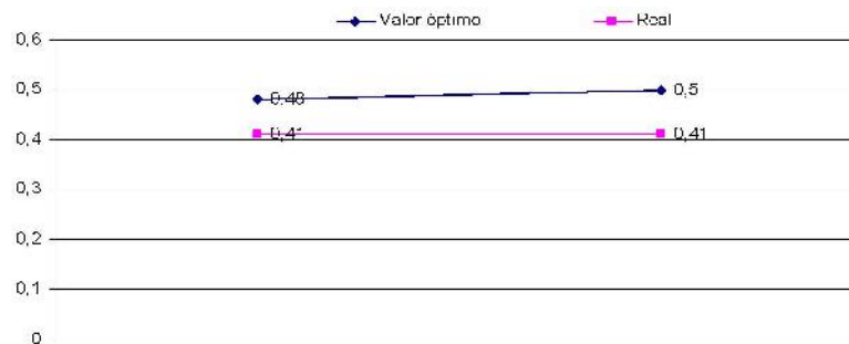
Gráfico 2. Valores óptimos del coeficiente de aprovechamiento del recorrido ( ).
